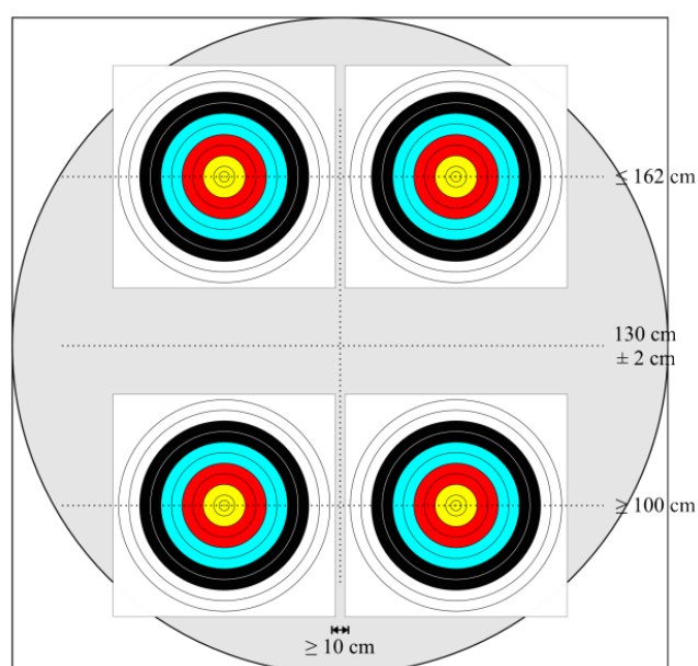
Disposizione 4 visuali triple per il Tiro alla Targa al Chiuso
