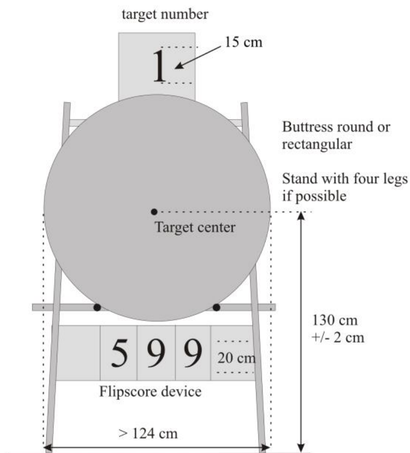
Disposizione 4 visuali da 40cm per il Tiro alla Targa al Chiuso
